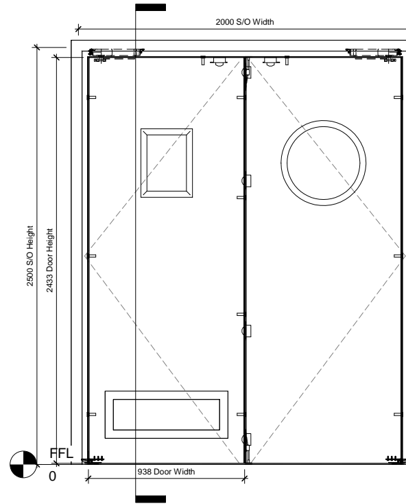
2 Door Elevation 1 : 20
